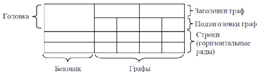
Рисунок 1 – Строение таблицы
